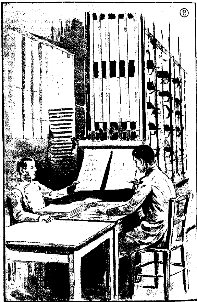
Machine à gommer et à sécher les timbres-poste. Côté où les feuilles sont reçues après leur évolution et où elles sont divisées par la cisaille circulaire.
