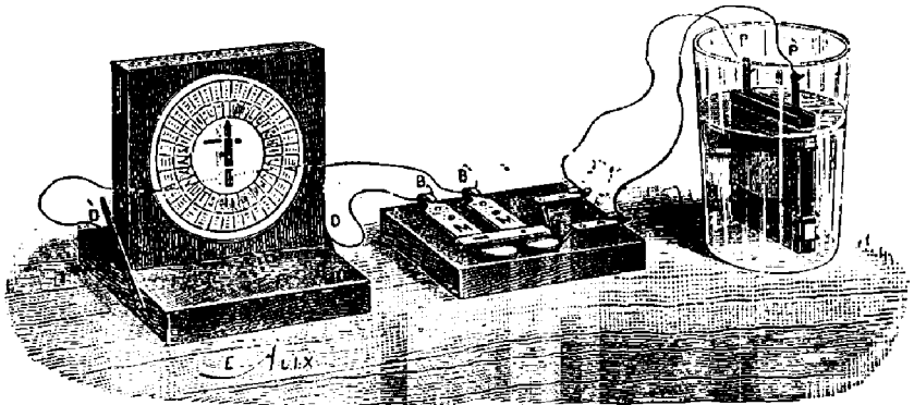
1° Télégraphe miniature, à signaux Morse, avec pile au sel et fils conducteurs 3 fr. 25 (port 0 fr. 85).
